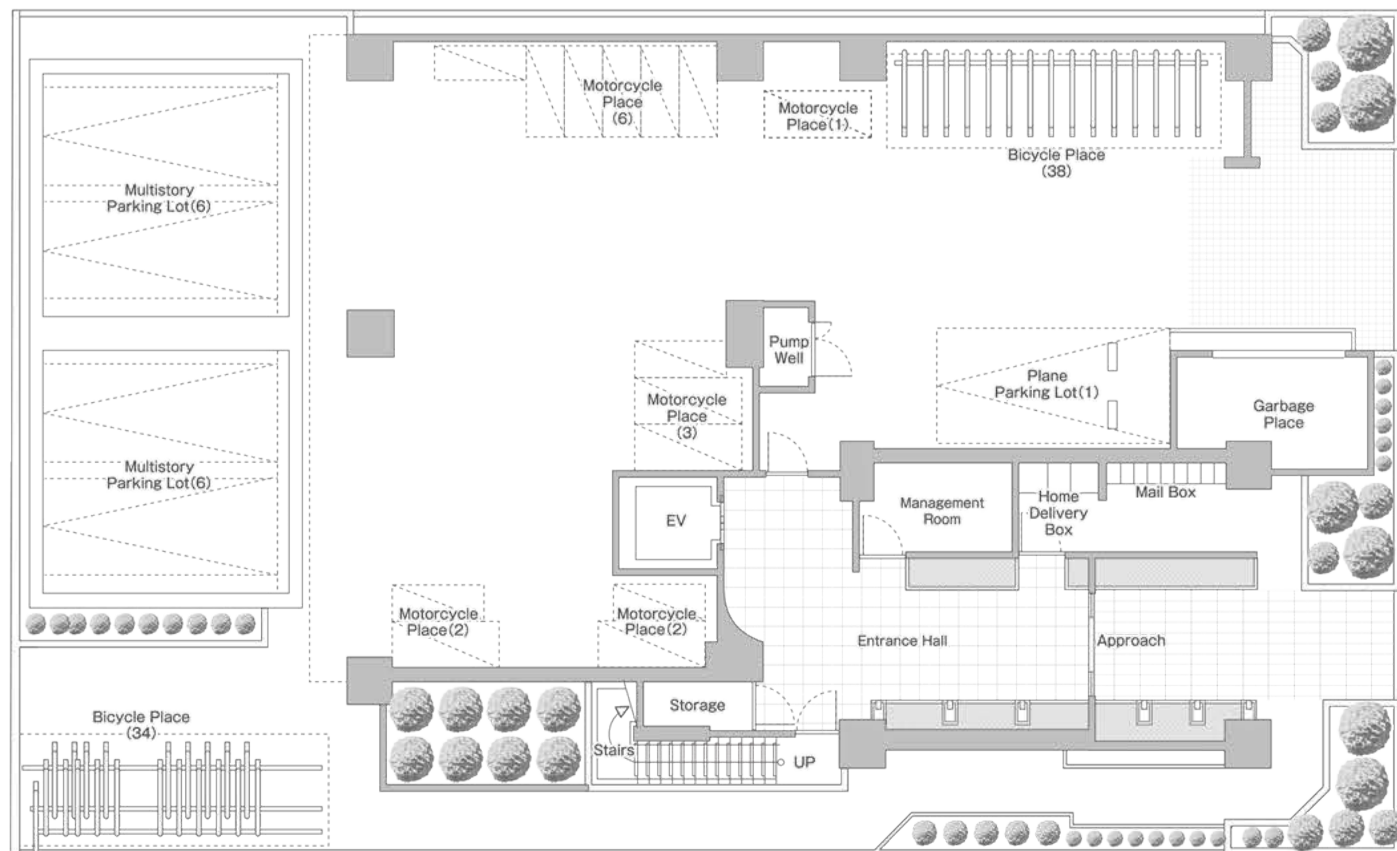
フロア平面図 1階
