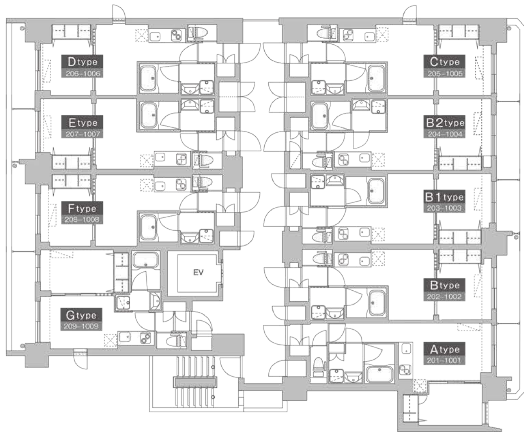
フロア平面図 2階-10階
